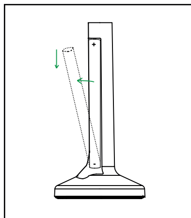
étape 5 : retirez la batterie. Exercez une pression sur la batterie, vers le bas, pour la retirer. Remarque: l'appareil doit être éteint avant de retirer la batterie.
